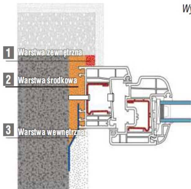
Uszczelnienie szczeliny między oknem a ościeżem
